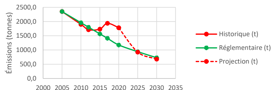
Evolution des émissions de NOx depuis 2005 et projetées à 2030 - CA Ardenne Métropole
