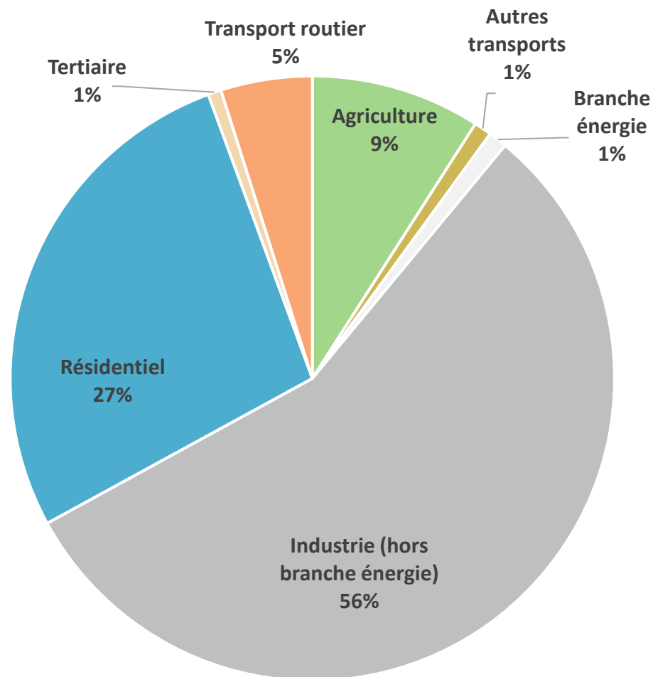
Répartition des émissions de PM 10 par secteur en 2020 - CA Ardenne Métropole
