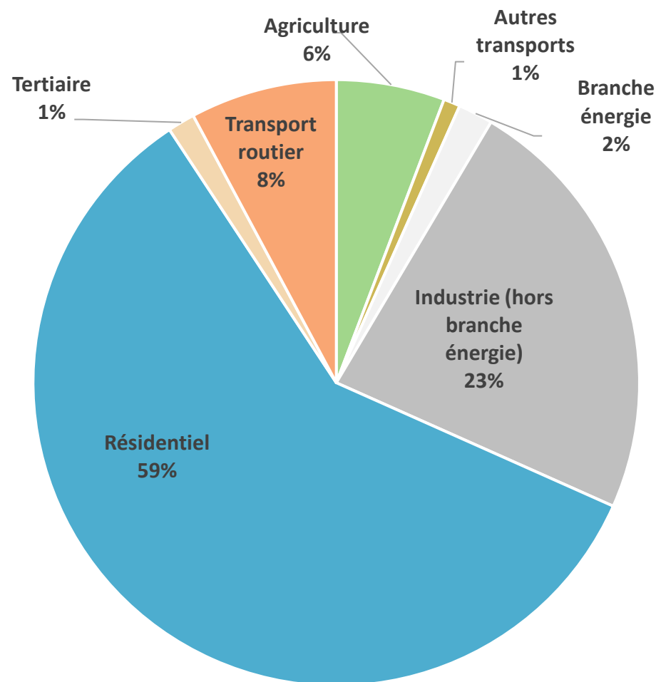
Répartition des émissions de PM 2,5 par secteur en 2020 - CA Ardenne Métropole
