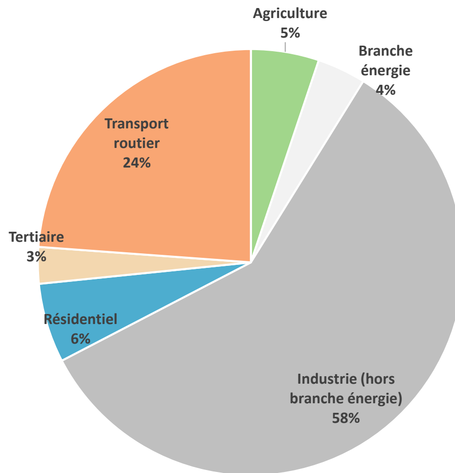
Répartition des émissions de NOx par secteur en 2020 - CA Ardenne Métropole
