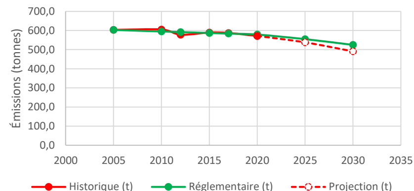
Evolution des émissions de NH 3 depuis 2005 et projetées à 2030 - CA Ardenne Métropole
