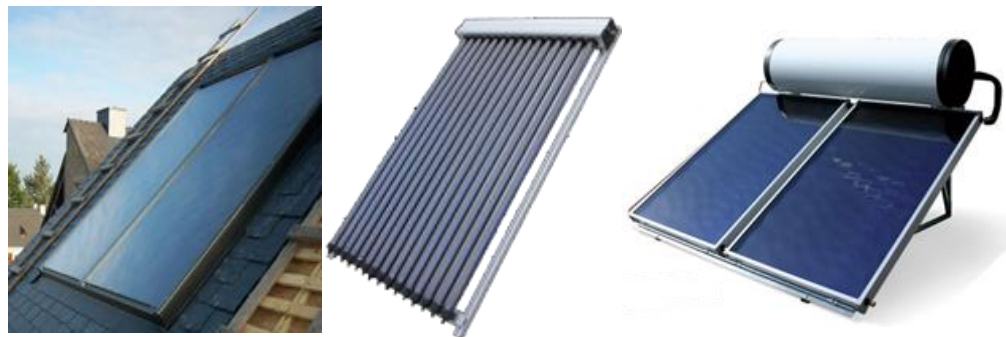
Différent systèmes solaires thermiques (de gauche à droite : capteur plan vitré, capteur tubulaire et monobloc)
