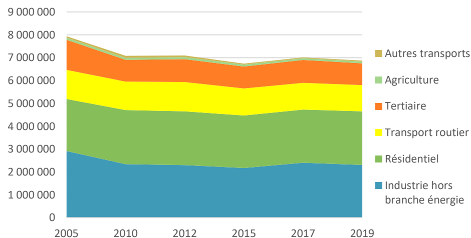
Evolution de la consommation d'énergie corrigée des variations climatiques par secteur entre 2005 et 2019 (MWh)
