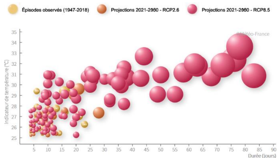
Fréquence et intensité des vagues de chaleur en Ardennes à l'horizon 2100
