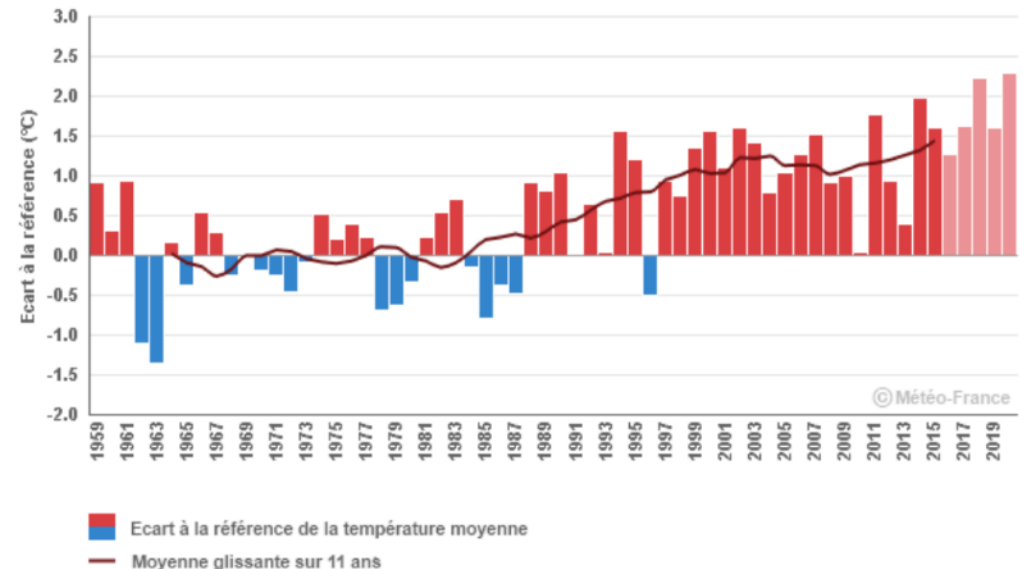
Températures moyennes annuelles : écart à la référence 1961 à 1990, Station Juniville
