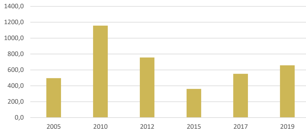
Evolution de la production de bois-énergie sur le territoire (GWh)
