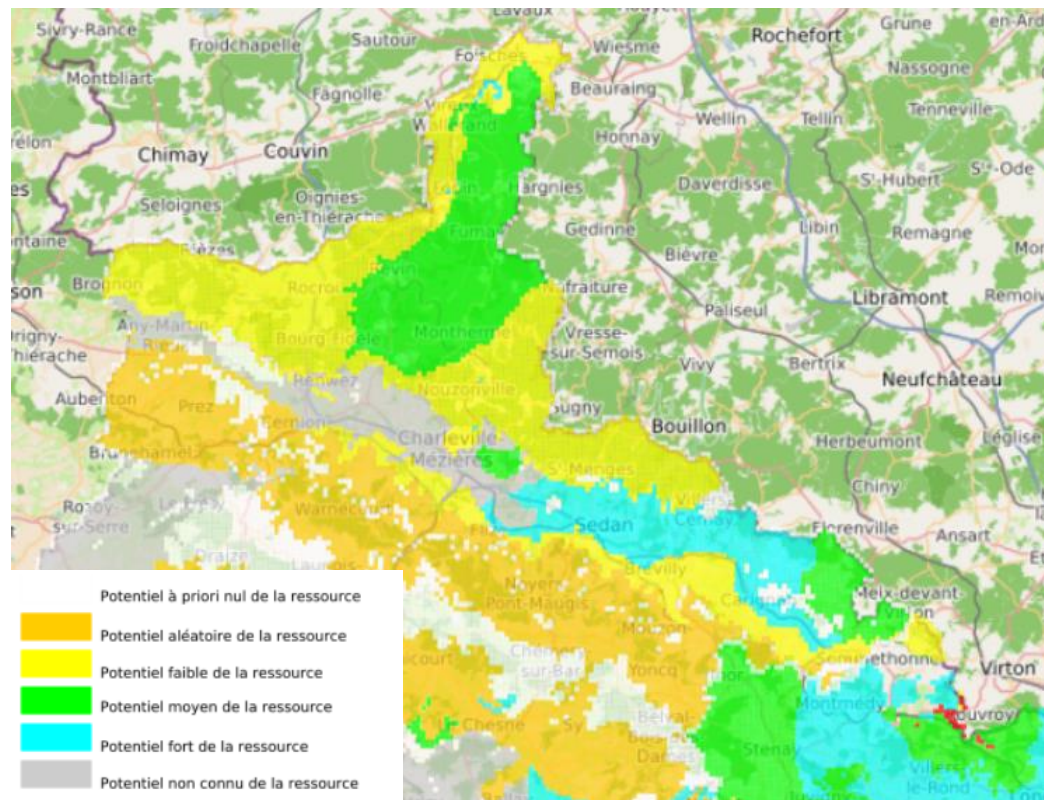
Ressources géothermiques de surface sur système ouvert (nappe)
