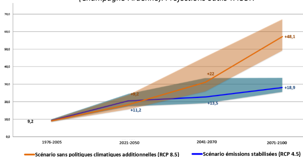
Anomalie du nombre de jours de vague de chaleur sur l'année entière (Champagne-Ardenne). Projections outils TACCT.
