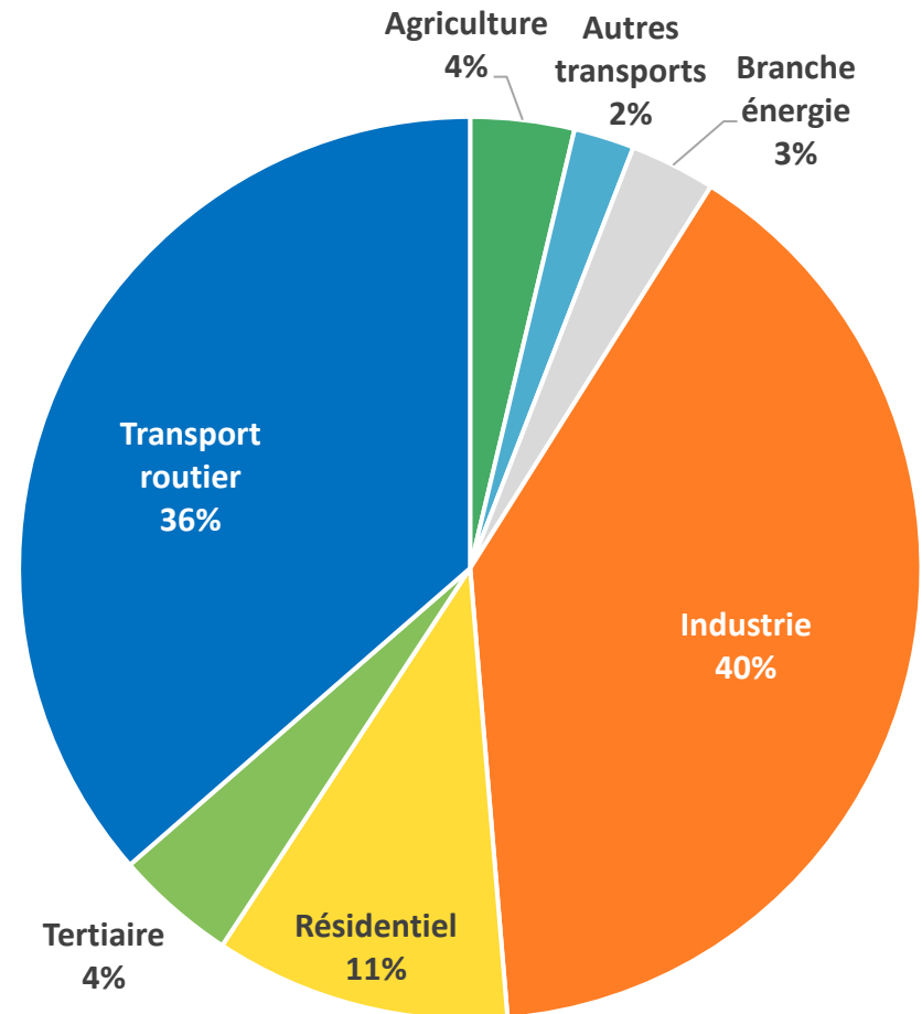
Emissions de NOx par secteur
