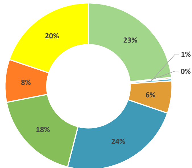
Répartition des émissions de gaz à effet de serre du territoire par secteur
